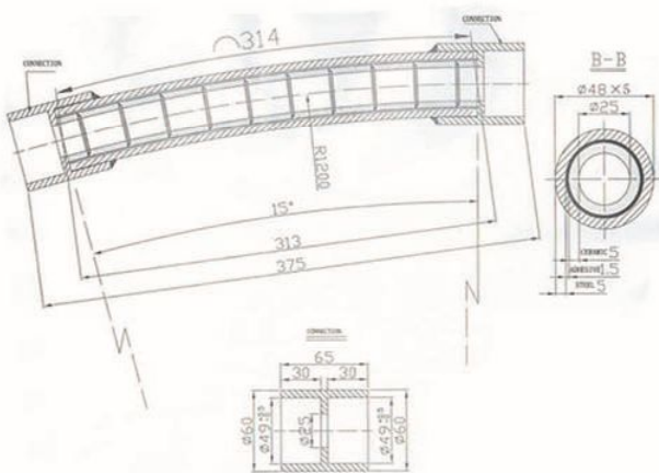
Pre-engineered Ceramics for Pipe Lining of Power Plant Pre - Engineered ceramicas de revestimiento de tubería para planta eléctrica
